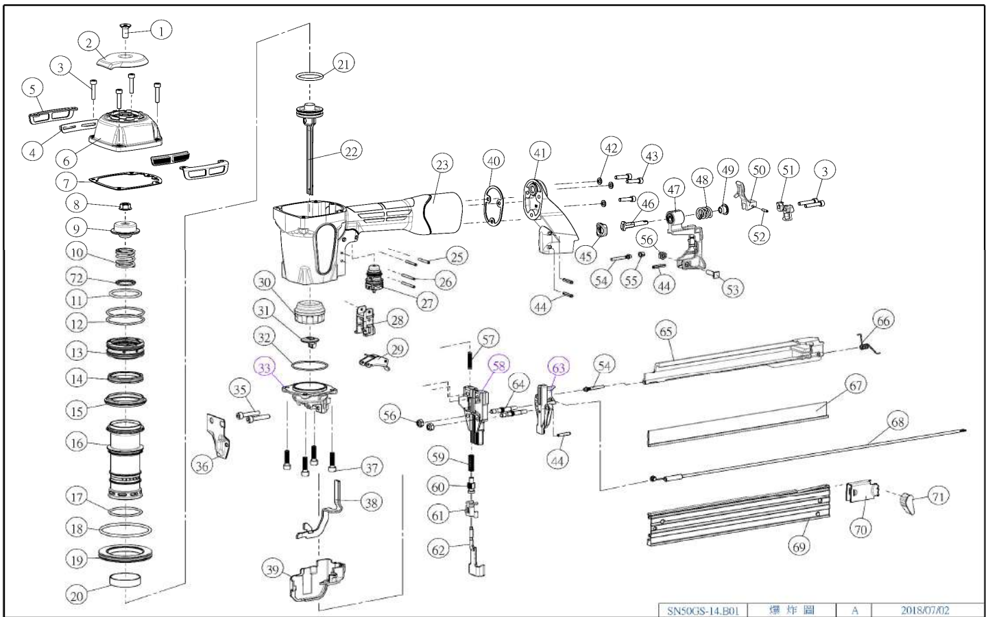
SN50GS-14.B01 爆炸圖 A 2018/07/02
