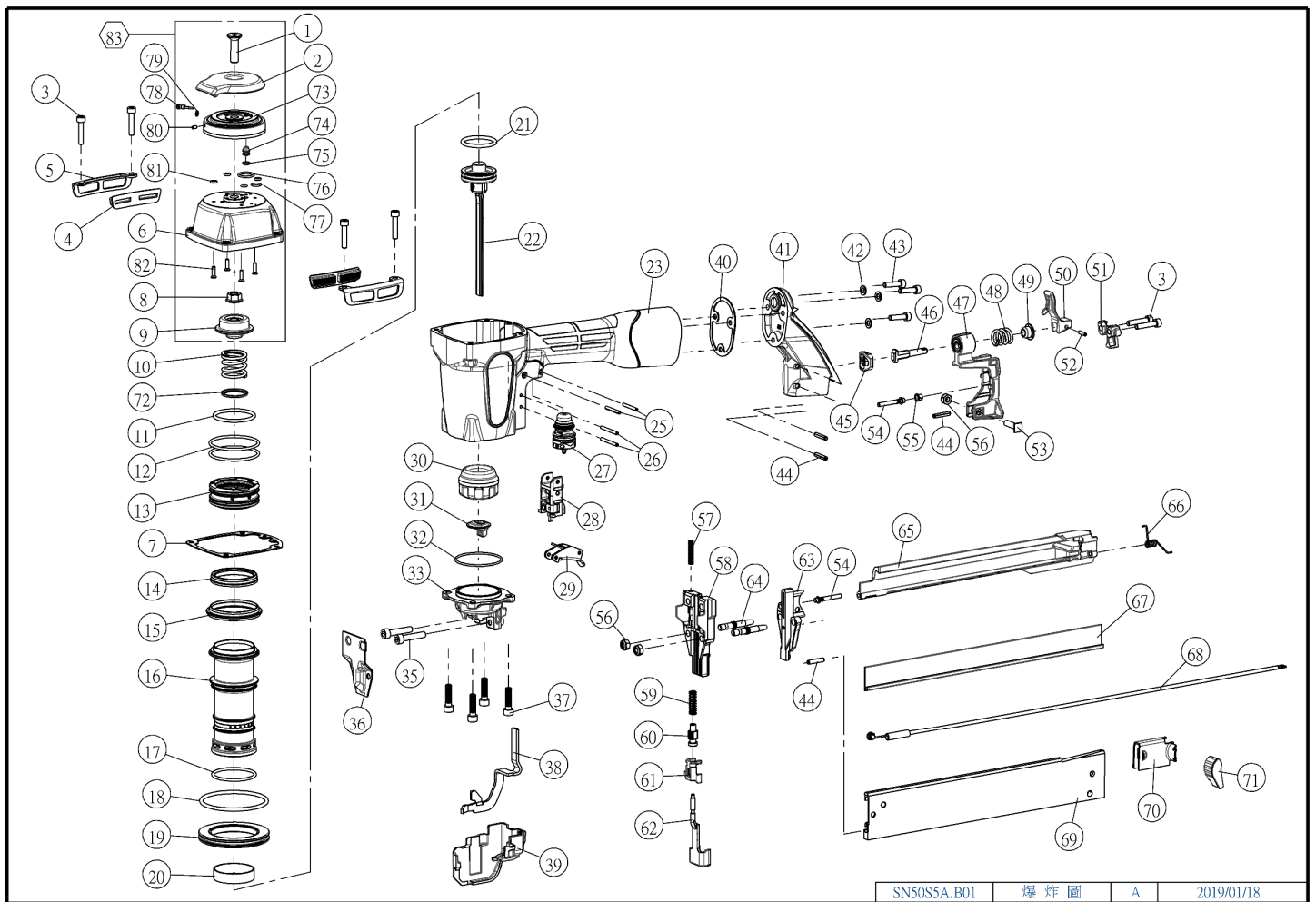
SN50S5A.B01 爆炸圖 A 2019/01/18
