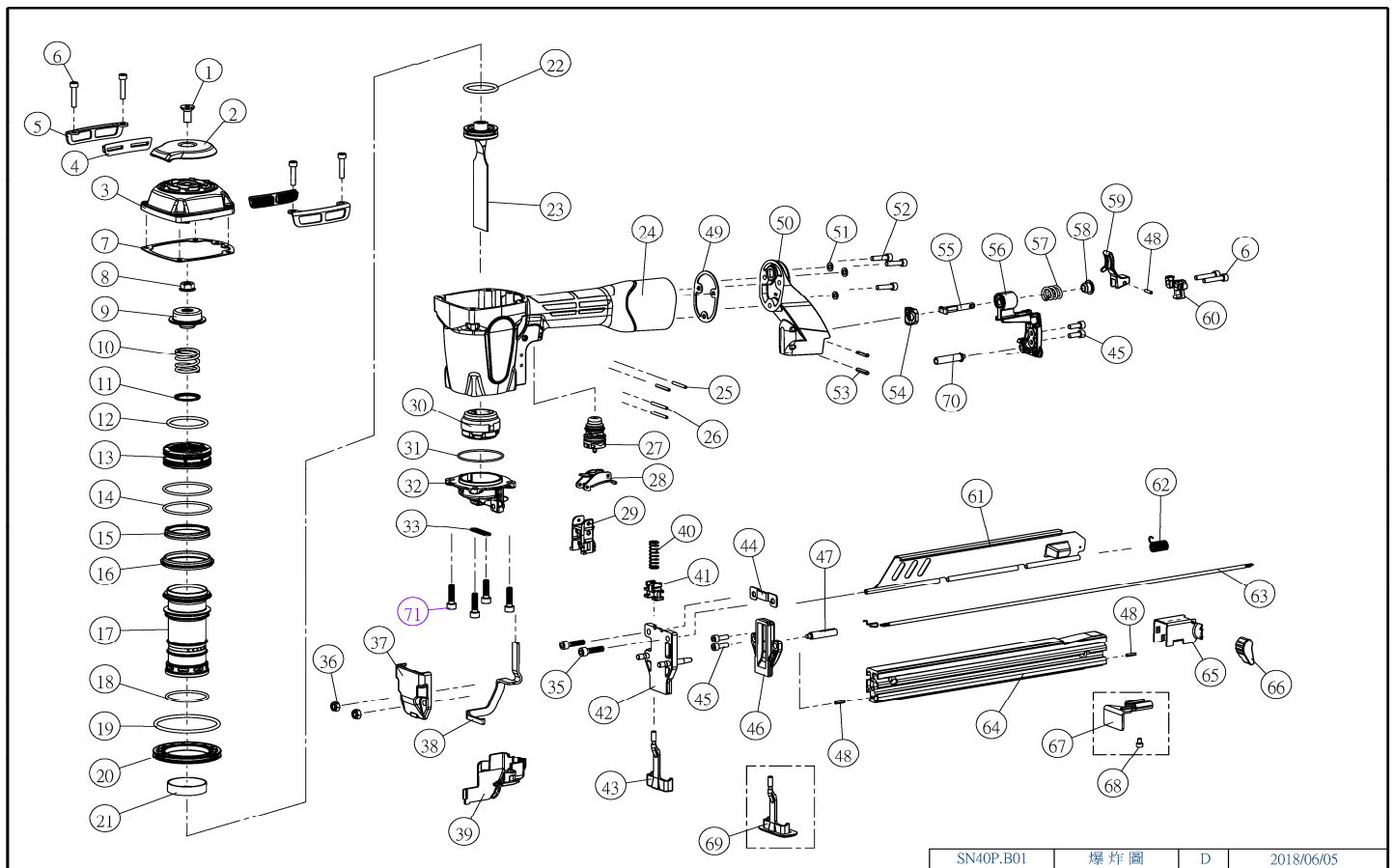
SN40P.B01 爆炸圖 D 2018/06/05
