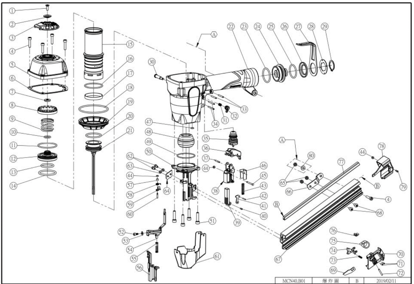
MCN40.B01 爆炸圖 B 2019/02/11
