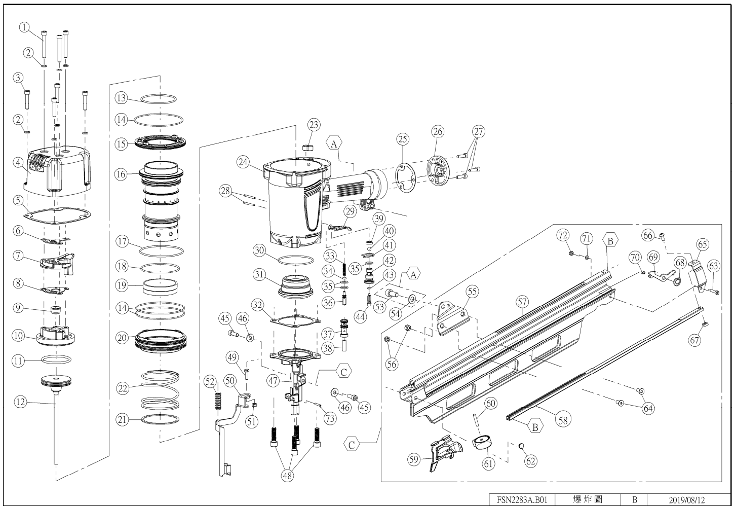
FSN2283A.B01 爆炸圖 B 2019/08/12
