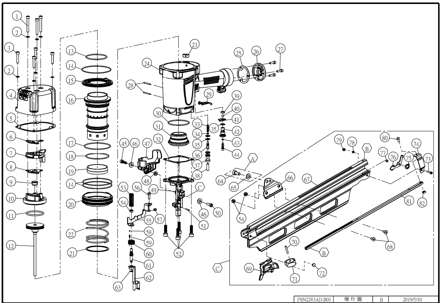
FSN2283AD.B01 爆炸圖 B 2019/5/10
