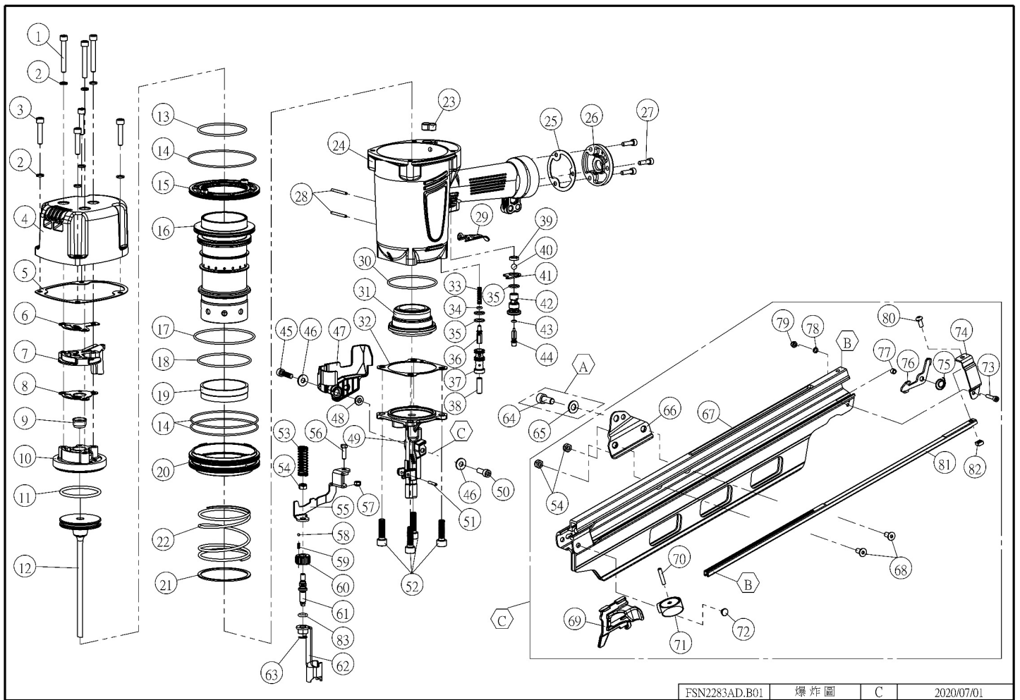
FSN2283AD.B01 爆炸圖 C 2020/07/01
